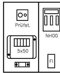
ESV Einschub 53 87kVA
