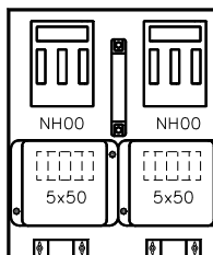
ESV Einschub 51 139kVA
