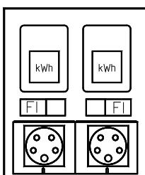
ESV Einschub 43-63 87kVA
