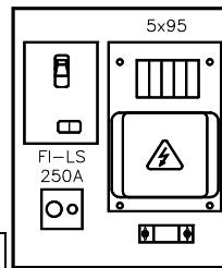
ESV Einschub 58 173kVA
